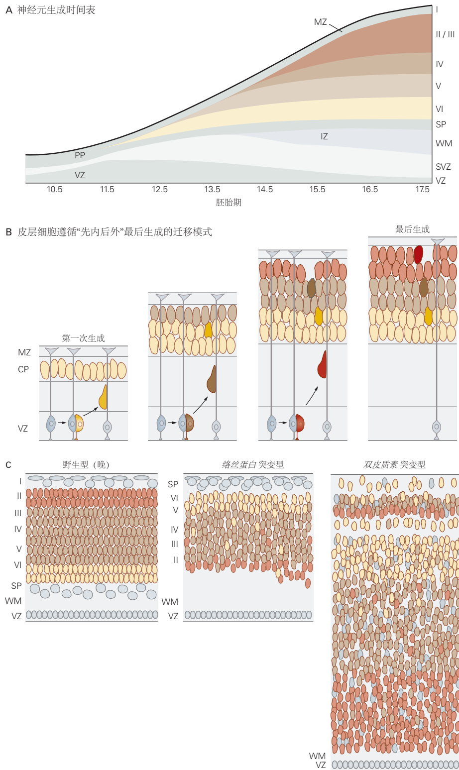
图 46.4.1: 胚胎大脑皮层内神经元的迁移导致分层皮质组织 [416] 。A. 这种神经发生的时间序列适用于小鼠大脑皮层。在胚胎发育的最后 5 天，神经元开始在皮层板中积累。在皮层板内，神经元在进入表层之前填充在深层。B. 在正常皮质发育过程中，神经元在进入皮层板时使用放射状胶质细胞作为迁移支架。当它们接近软膜表面时，神经元停止迁移并从放射状神经胶质细胞中分离出来。这种由内而外有序的神经元迁移模式导致成熟大脑皮层中形成 6 个神经元层，排列在白质和亚板之间。C. 在缺乏功能性络丝蛋白的小鼠突变络丝蛋白中，皮层板中神经元的分层被严重破坏并部分倒置。此外，整个皮层板在亚板下方发育。在双皮质素突变体中，皮层变厚，神经元失去其特征性的分层特性，并且某些层包含更少的神经元。在 Lis1 基因突变体中观察到类似的破坏，这是某些形式的人类无脑畸形的基础。
