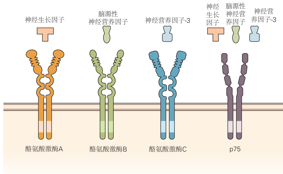
图 46.8.5: 神经营养因子及其受体。3 种主要神经营养蛋白中的每一种都与不同的跨膜酪氨酸激酶相互作用。此外，所有 3 种神经营养蛋白都可以与低亲和力神经营养蛋白受体 p75 结合 [421] 。
