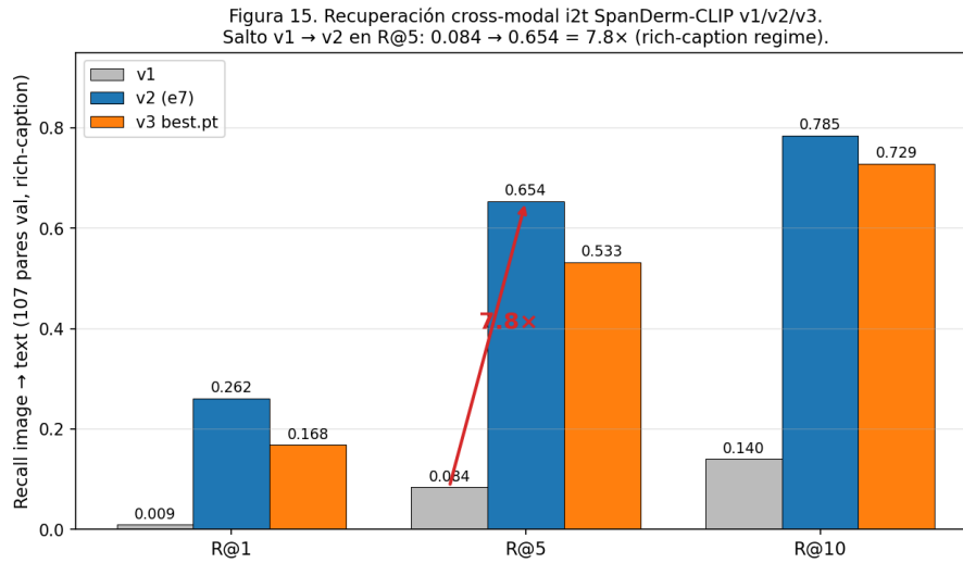
Figura 4.11: Recuperación cross-modal i2t R@5 de la rama contrastiva de Dermapixel R0 sobre 107 pares de validación, régimen rich-caption . Pico v2 de 14,0× de lift sobre el azar (0,047 → 0,654) atribuible al conjunto LoRA textual + captions sintéticas ricas generadas mediante un modelo de lenguaje grande. v4 y v5 conservan lift sustancial (12,4× y 10,8× respectivamente) pero descienden respecto al pico, en coherencia con la degradación documentada sobre el régimen híbrido.
