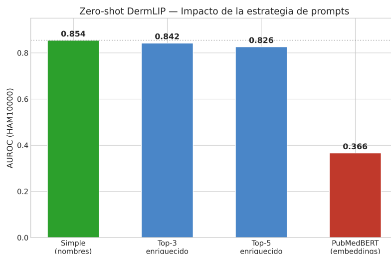
Figura 4.7: Sensibilidad zero-shot al tokenizador y a la formulación del prompt sobre HAM10000. La AUROC oscila entre 0,366 (DermLIP v1/v2 + PubMedBERT + prompts genéricos) y 0,854 (DermLIP original + GPT-2/CLIP + prompts A3 de Derm1M), un rango de 48,8 pp para variaciones que no afectan al encoder visual.
