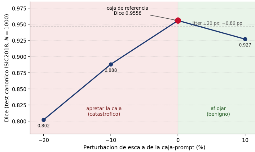
Figura 4.6: Robustez de MedSAM2-tiny a la calidad de la caja- prompt sobre el test canónico de ISIC2018 ( N = 1000 ). El jitter de esquinas es prácticamente inocuo ( -0,86 pp), pero la escala es crítica y asimétrica: apretar la caja degrada mucho más que aflojarla.
