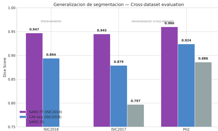
Figura 4.5: Segmentación binaria de lesión. SAM2.1-Large con fine-tuning del decodificador alcanza Dice 0,947 sobre ISIC2018, +2,6 pp sobre el resultado publicado por Yan et al. [1], con transferencia OOD prácticamente nula sobre ISIC2017 (0,945) y PH2 (0,960).
