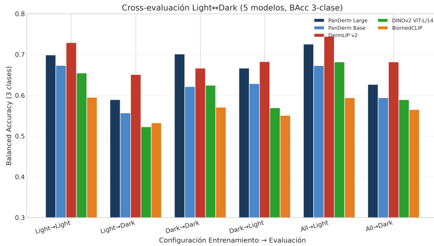
Figura 4.10: Evaluación cruzada Light ↔ Dark sobre Fitzpatrick17k (BAcc en formulación de tres clases). La caída L→D vs L→L cuantifica la pérdida de rendimiento al entrenar sólo con fototipos claros y evaluar sobre fototipos oscuros, máxima en DINOv2 ( \Delta = -0,132 pp).
