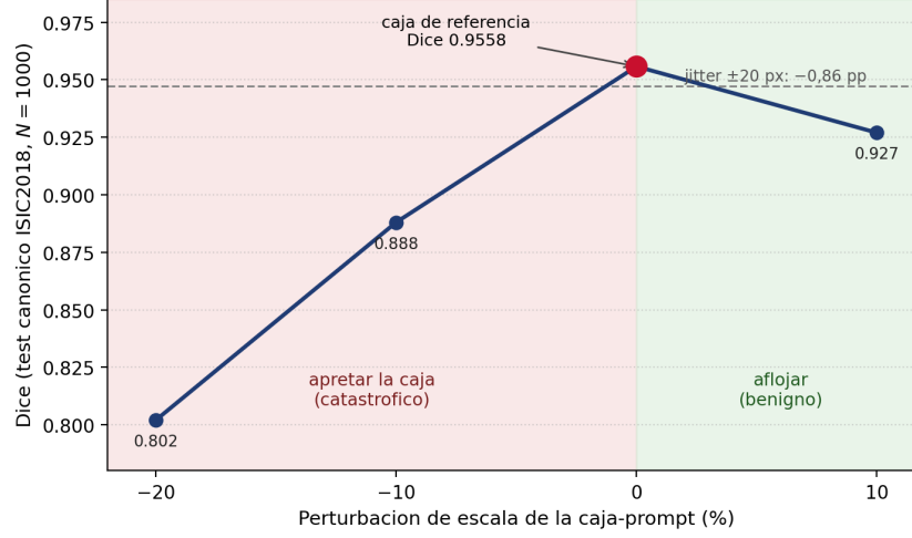
Figura 4.2: Robustez de MedSAM2-tiny a la calidad de la caja- prompt sobre el test canónico de ISIC2018 ( N = 1\,000 ). El jitter de esquinas es prácticamente inocuo (−0,86 pp), pero la escala es crítica y asimétrica: apretar la caja degrada mucho más que aflojarla.
