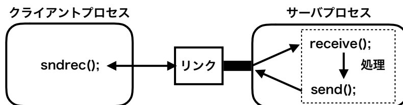
図 21.1: TacOS のメッセージ通信
