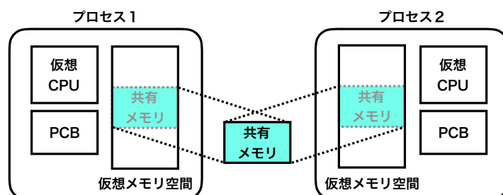
図 6.1: 共有メモリ
