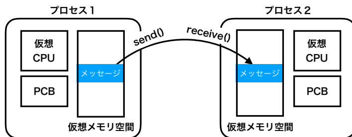
図 6.4: メッセージ通信
