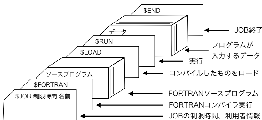
図 1.5: ジョブの構成
