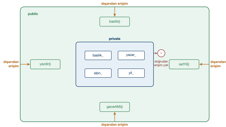
Şekil 3.1: Kapsülleme: private veri çekirdeği, yalnızca public arayüz kabuğu üzerinden erişilebilir olur.
