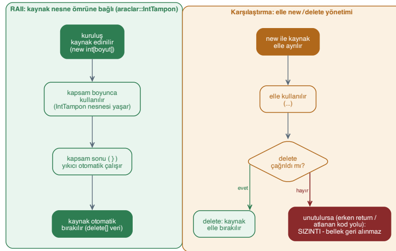
Şekil 2.3: RAII: kaynağın edinimi nesnenin kuruluşuna, bırakılması kapsam sonuna bağlanır. Elle yönetimde delete unutulursa yol sızıntıyla biter.
