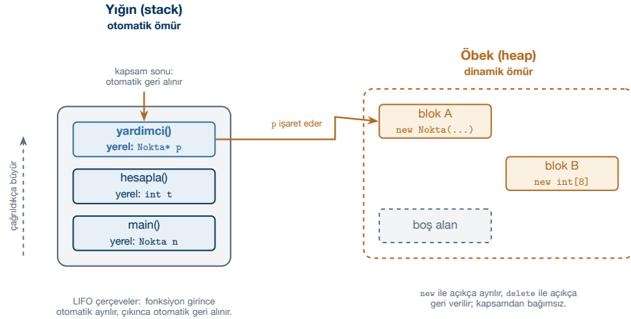
Şekil 2.2: Yığın (stack): kapsamla otomatik ayrılıp geri alınan çerçeveler. Öbek (heap): new/delete ile açıkça yönetilen, kapsamdan bağımsız bloklar.
