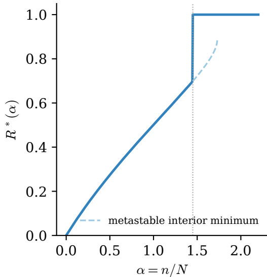
order parameter jumps ( \varepsilon: 0.25 \rightarrow 0 )
