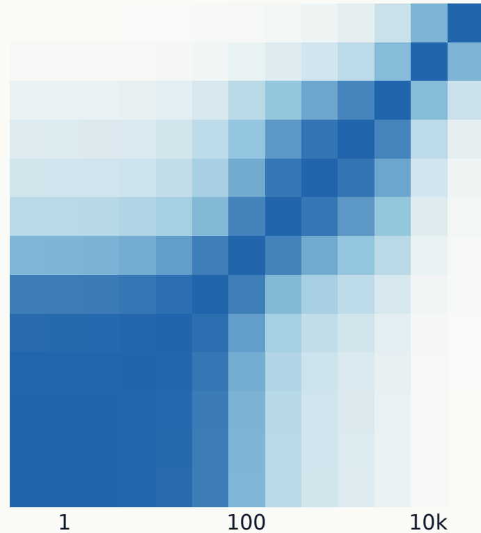
Gaussian · Tensor
