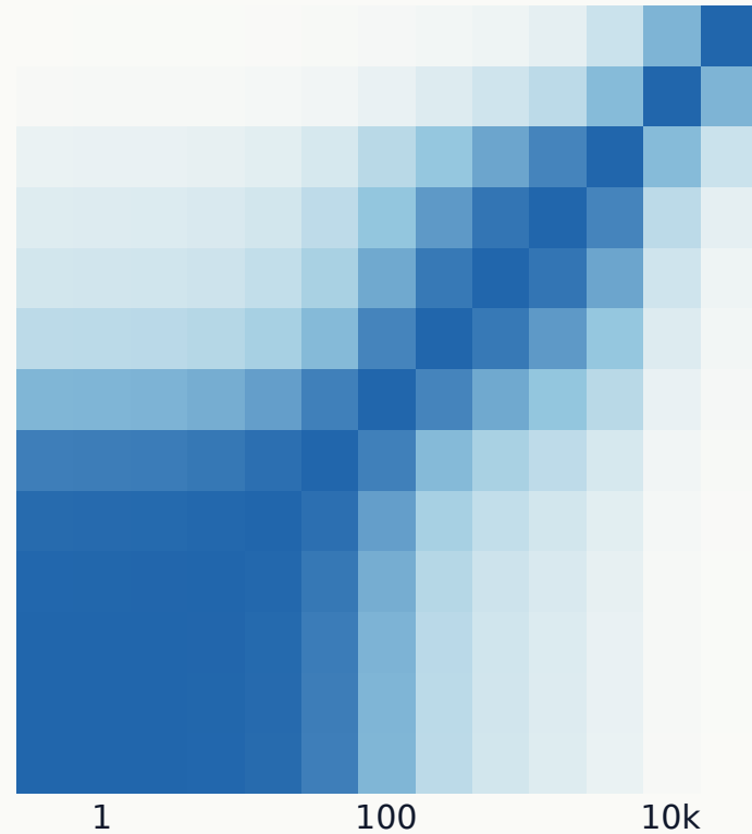
Gaussian · logits
