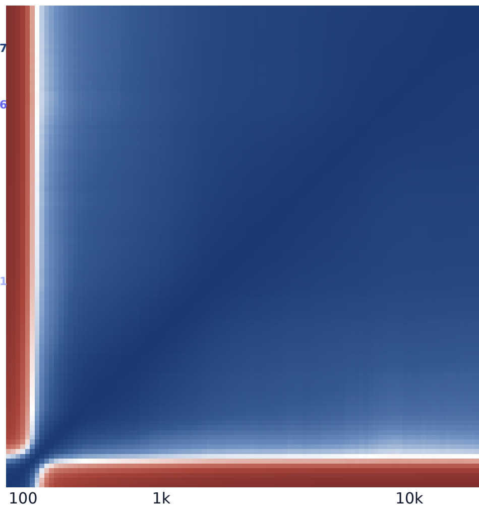
Gaussian · logits
