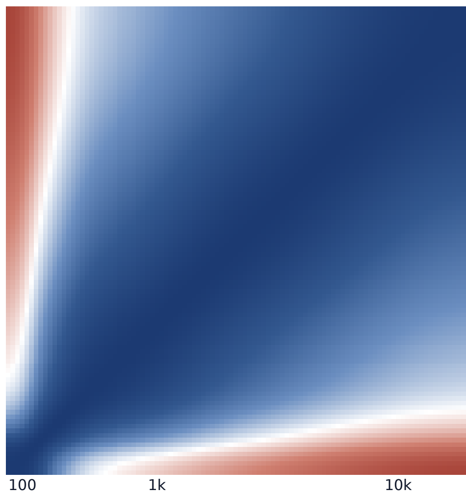
Gaussian · logits
