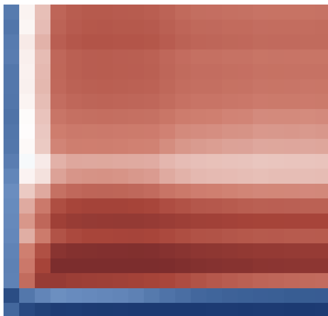
layer1
