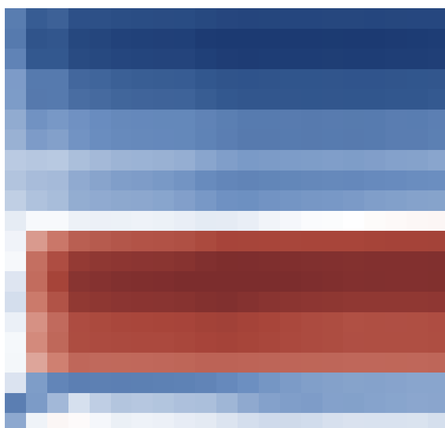
layer2
