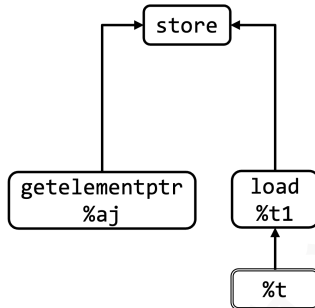
(c) 指令选择子图 2
