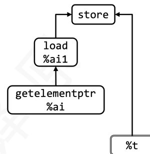
(d) 指令选择子图 3
