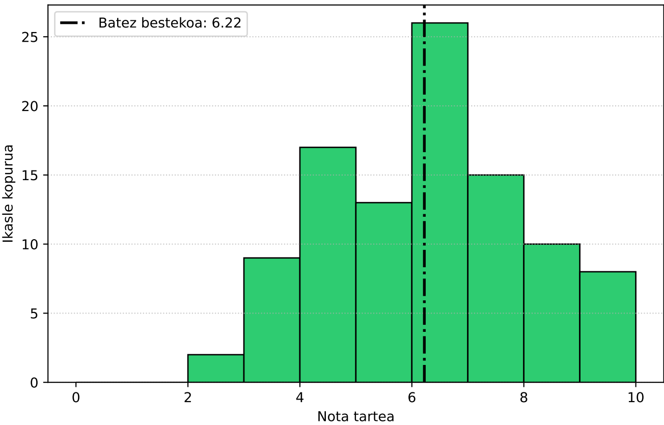
3. Noten Maiztasun-Banaketa (100 ikasle)
