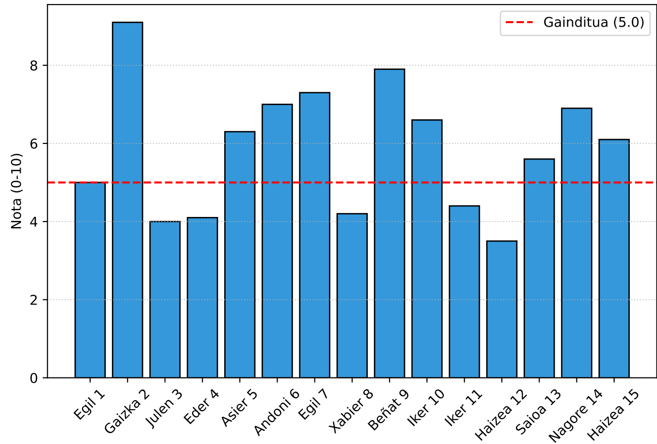
1. Ikasleen Notak (Lehen 15 ikasle)
