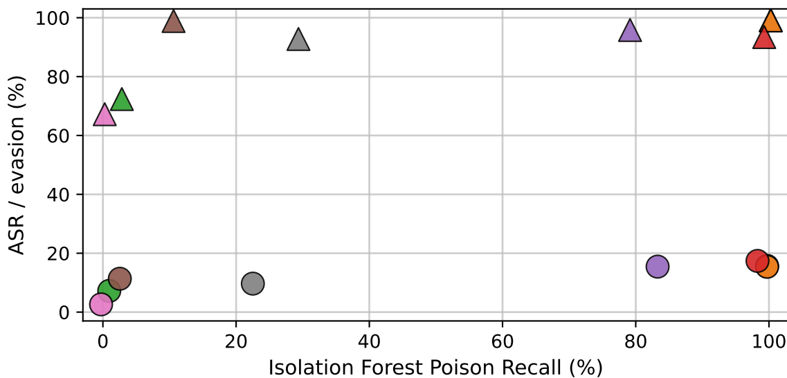
EMBER 2024 Win64
