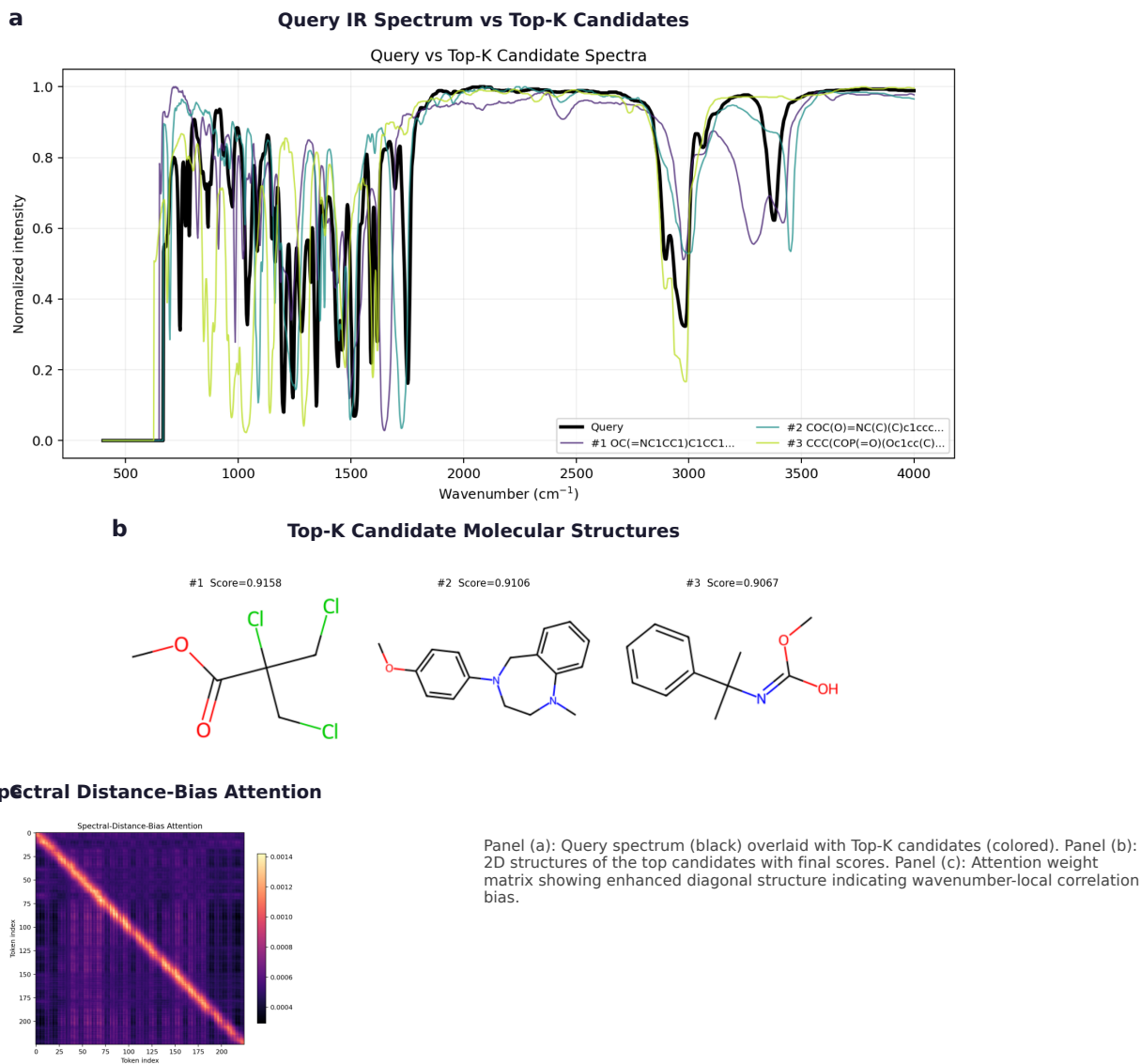
图 2: Demo 输出示例。(a) 查询光谱（黑色）与 Top-K 候选（彩色）叠加对比。(b) Top-K 候选分子二维结构及得分。(c) 谱图距离偏置注意力热图，对角线增强表明波数邻近区域具有更强局部相关性。
