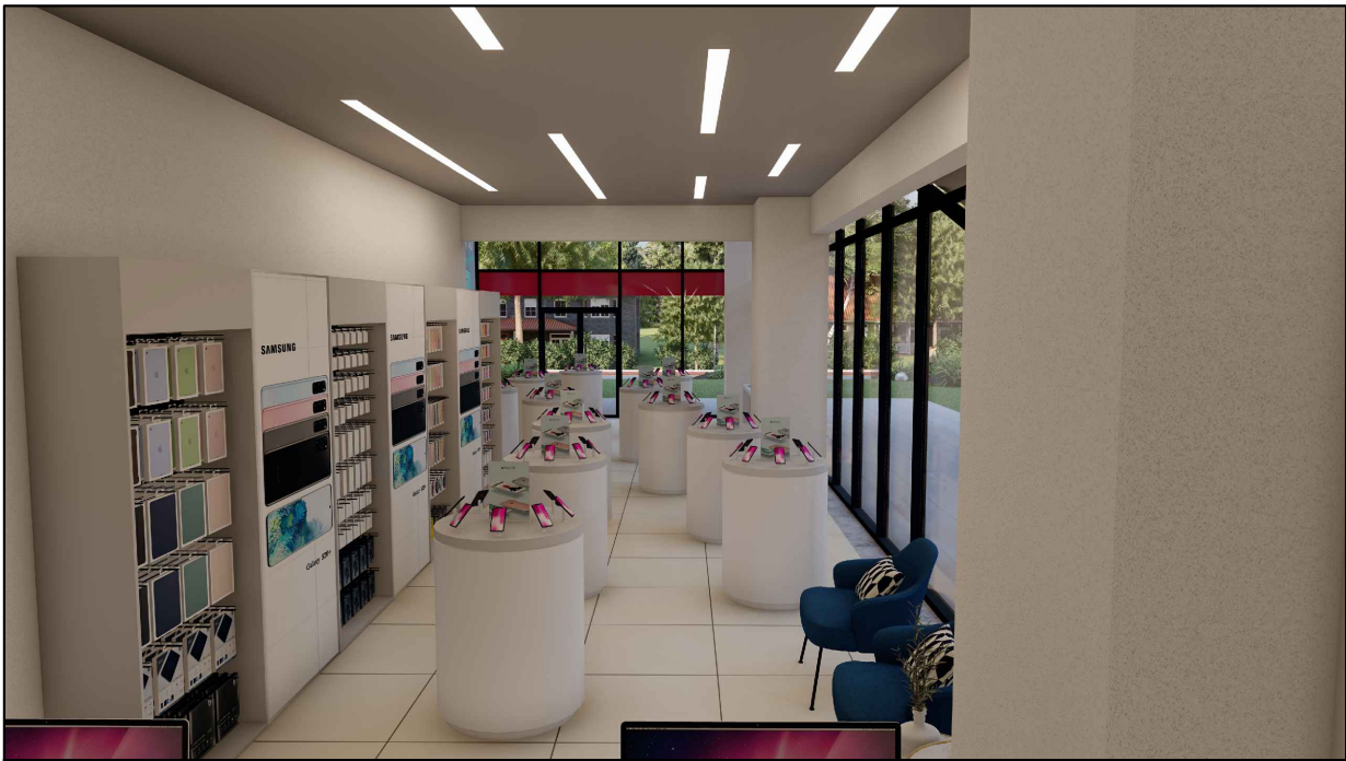
2 IMAGEM RENDERIZADA ESCALA: 1/100 OBS.: CONFERIR COTAS NA OBRA
