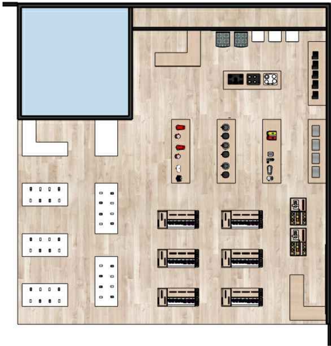
1 PLANTA BAIXA GERAL ESCALA: 1/100 OBS.: CONFERIR COTAS NA OBRA
