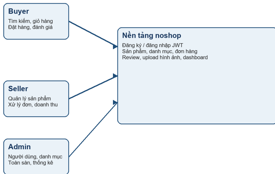
Hình 2.1. Tác nhân và các chức năng chính của noshop
