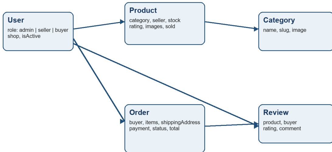
Mô hình dữ liệu MongoDB
