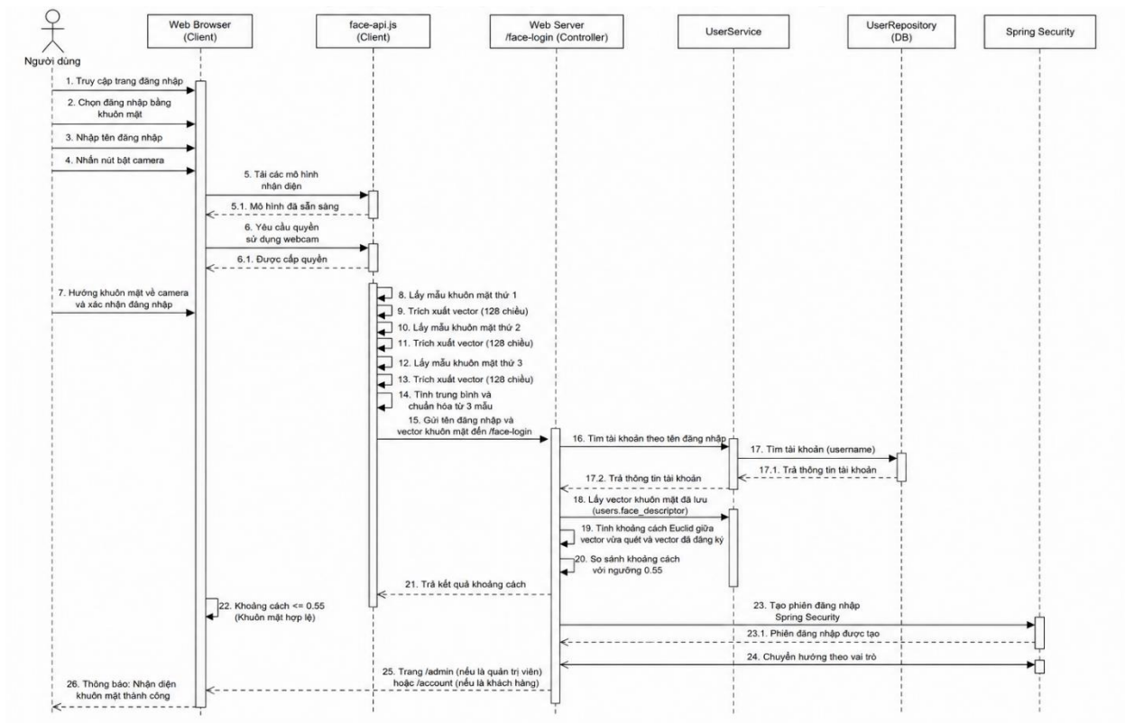
Hình 2.4. Sơ đồ tuần tự đăng nhập bằng khuôn mặt
