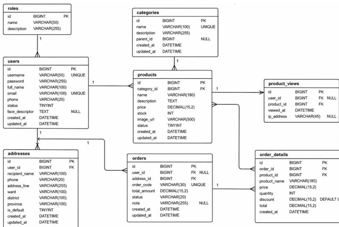
Hình 2.6. Sơ đồ quan hệ cơ sở dữ liệu của hệ thống
