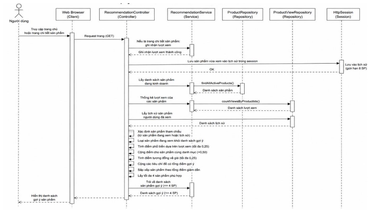
Hình 2.5. Sơ đồ tuần tự gợi ý sản phẩm
