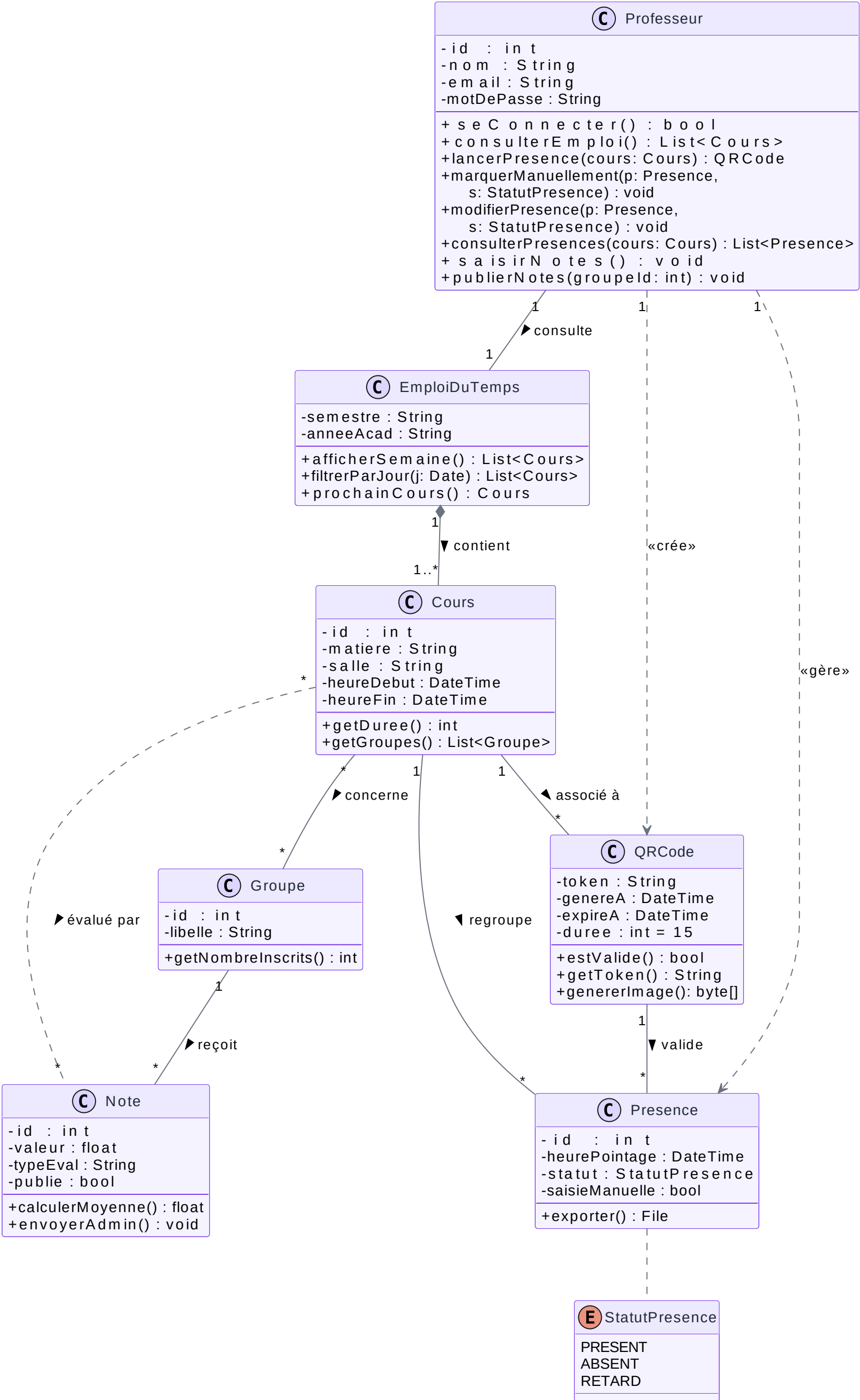
Diagramme de Classes — Espace Professeur
