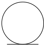
Database
