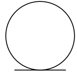
Database
