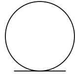
Database
