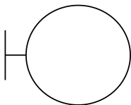
Login UI
