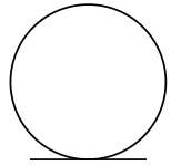
Database
