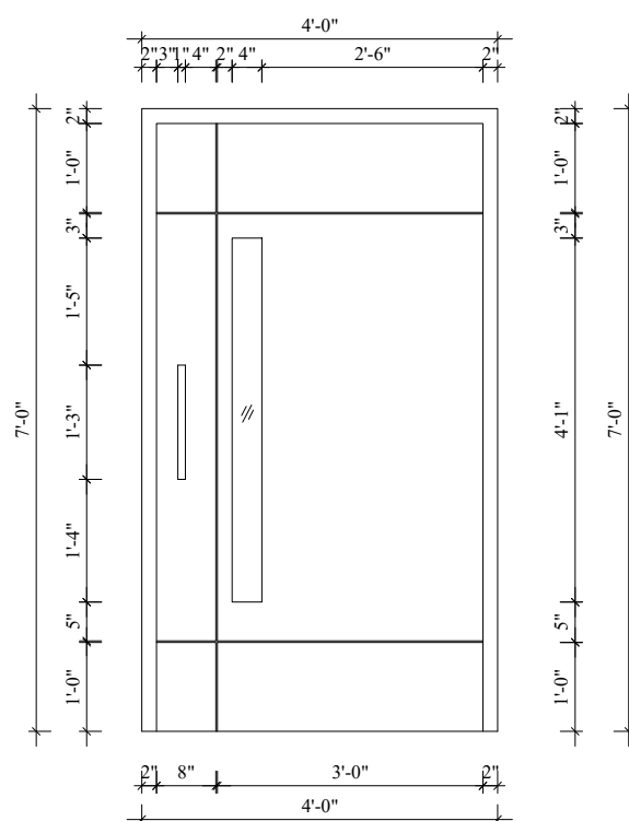
DOOR4 (D4)
