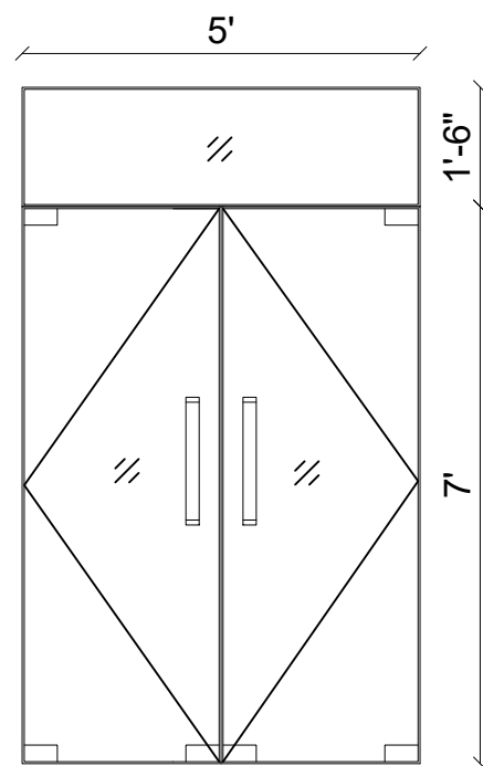
DOOR (D)
