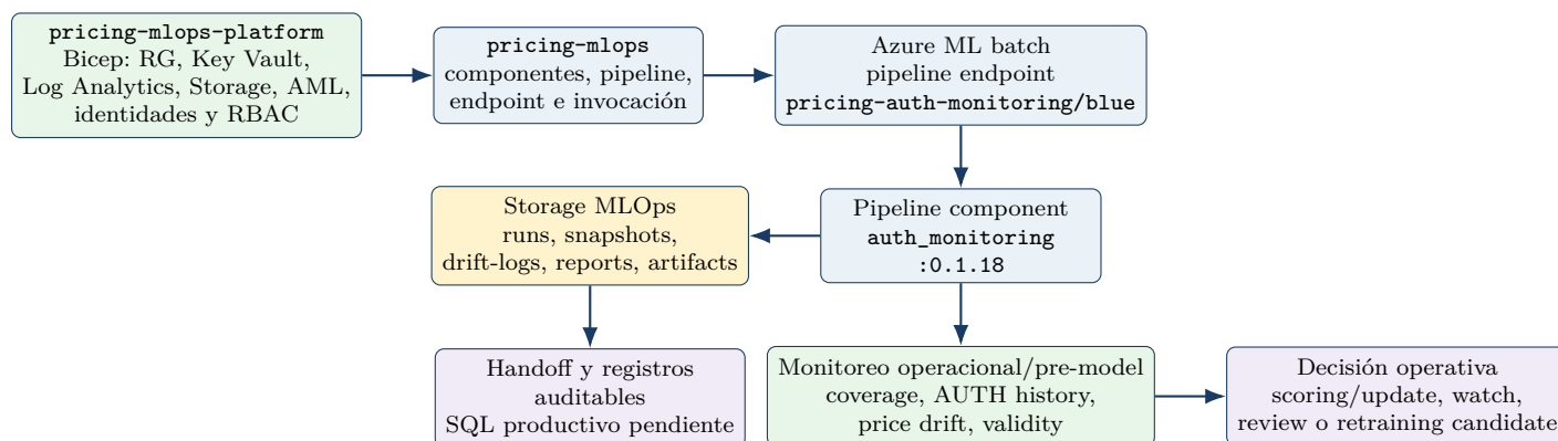
Figura 2: Arquitectura ejecutiva vigente de la solución en Azure.
