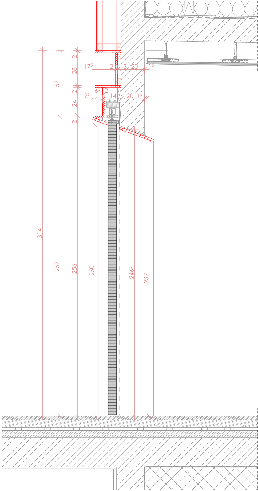
Coupe 2
