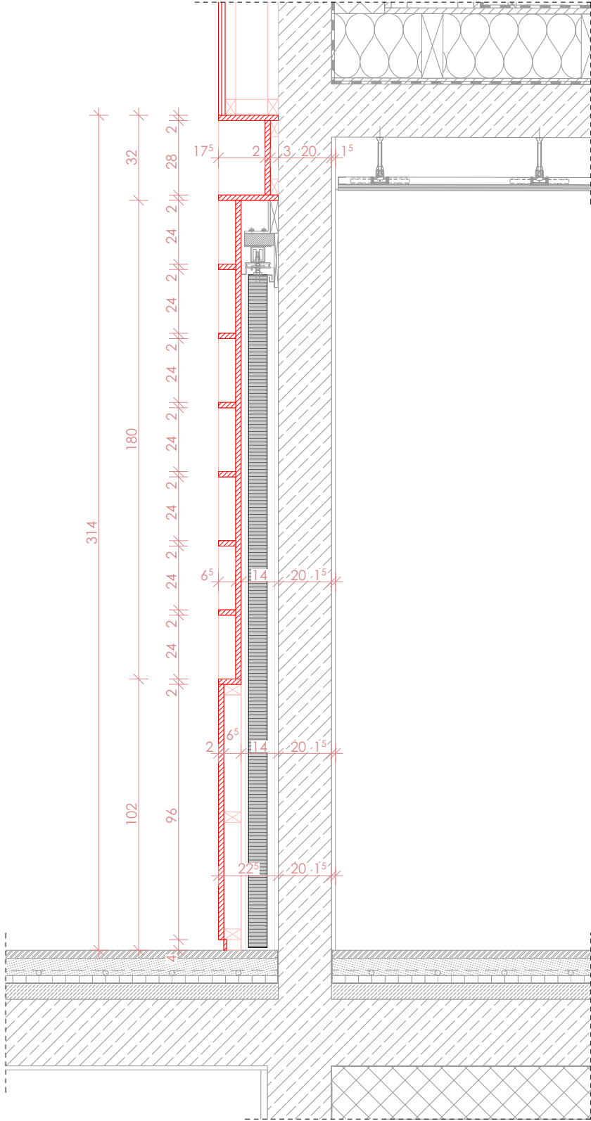
Coupe 3
