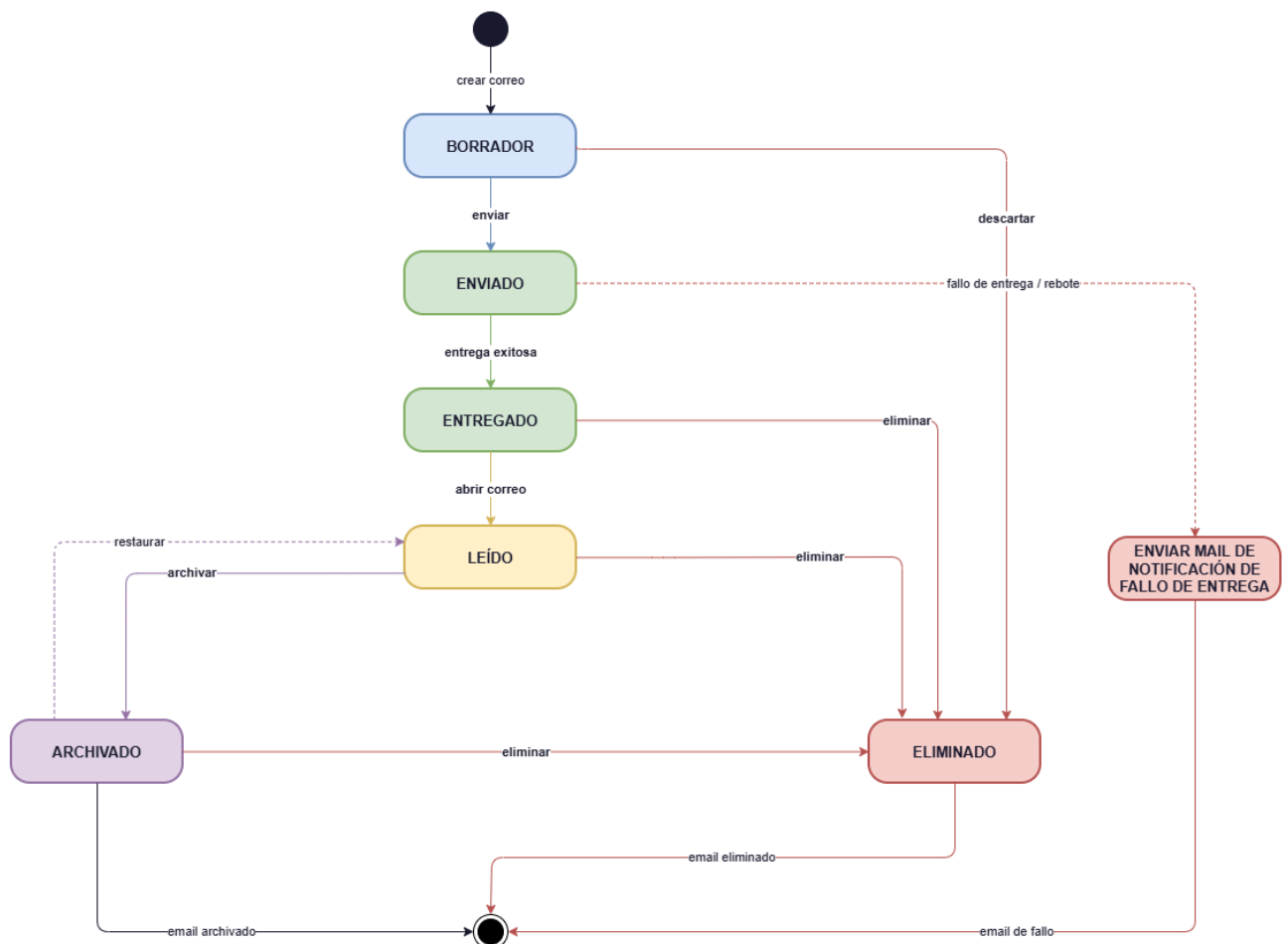
Diagrama de Estados — Ciclo de Vida de un Correo Electrónico
