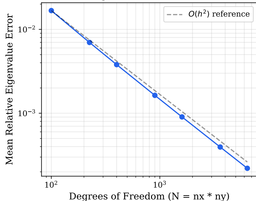
FDFD Eigenvalue Error vs Grid Size
