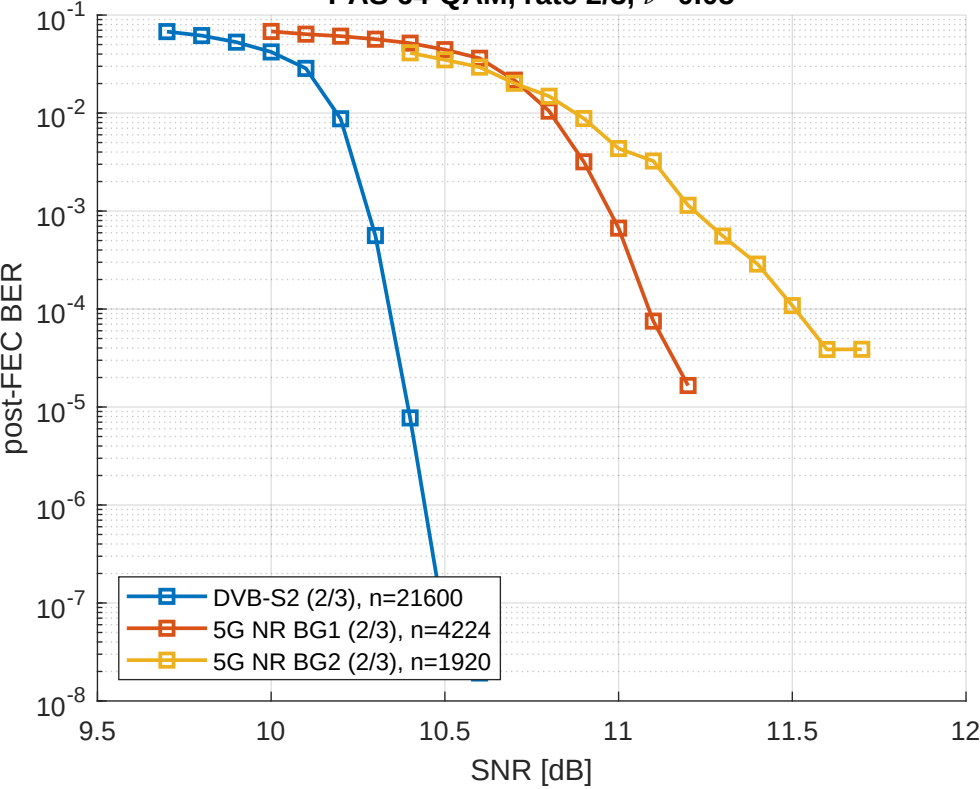
PAS 64-QAM, rate 2/3, \nu=0.05
