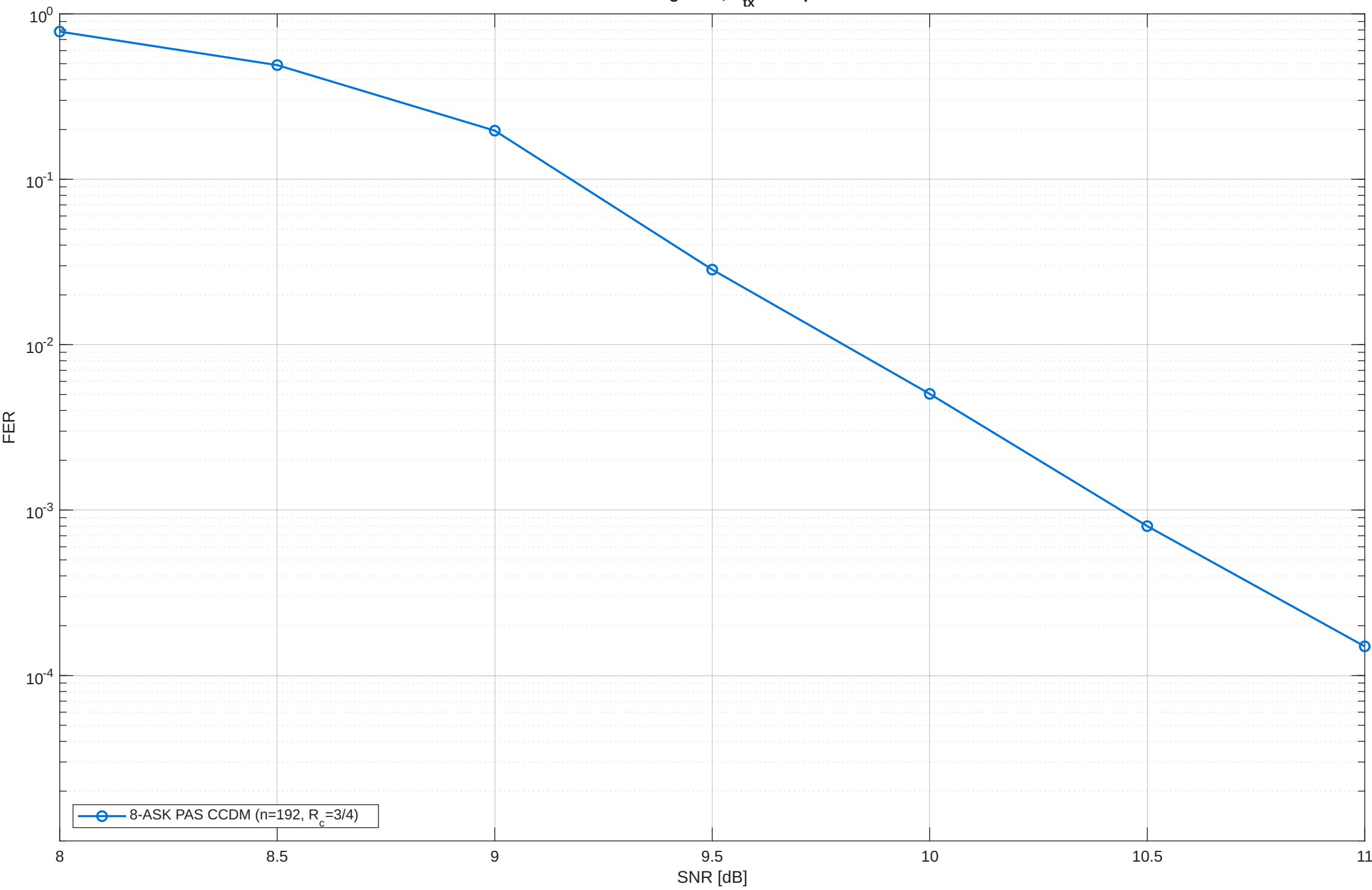
Steiner Fig. 3.32, R_{tx}=1.5 bpcu
