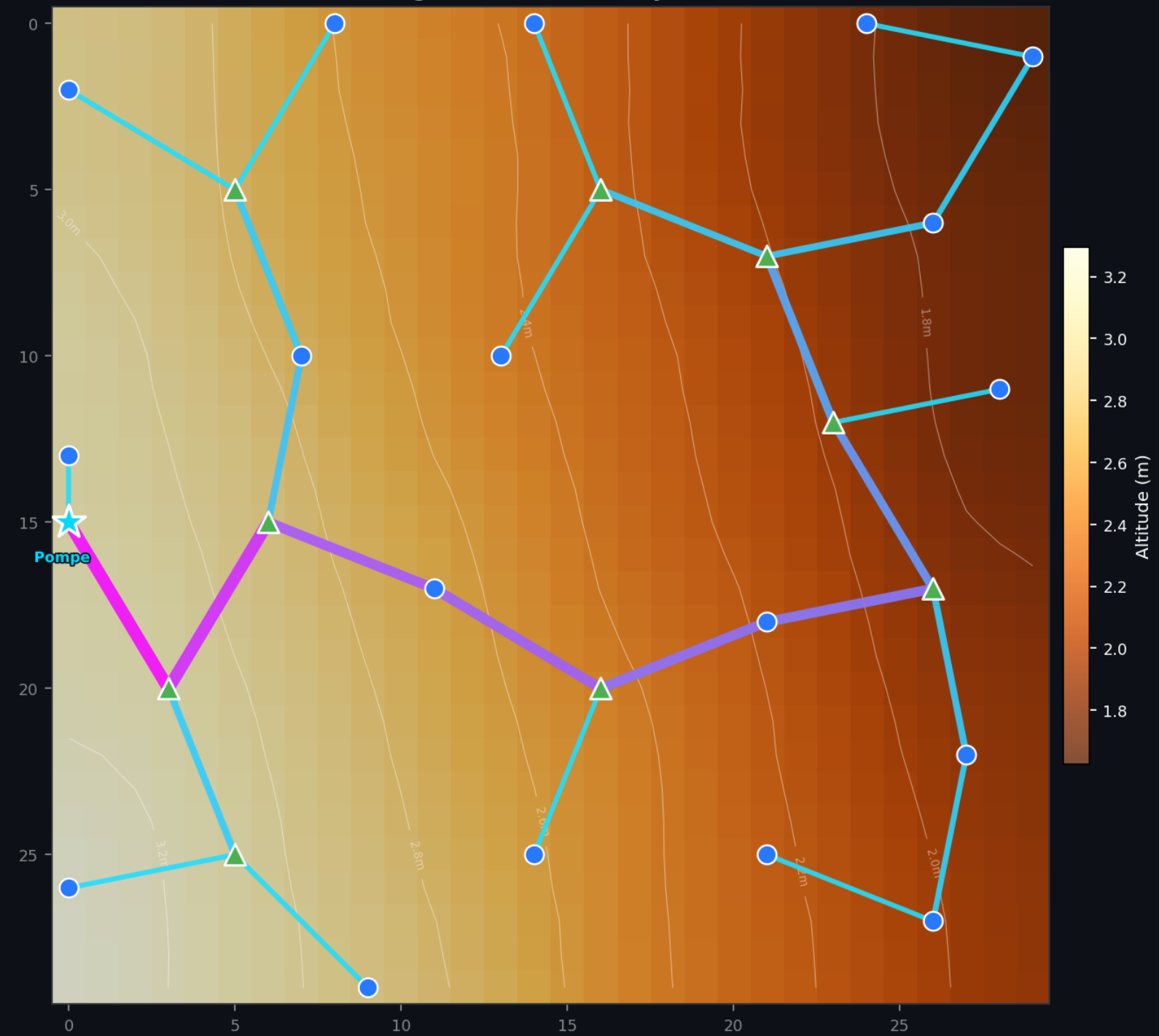
Relief — 150x150 m Lignes de niveau + tuyaux
