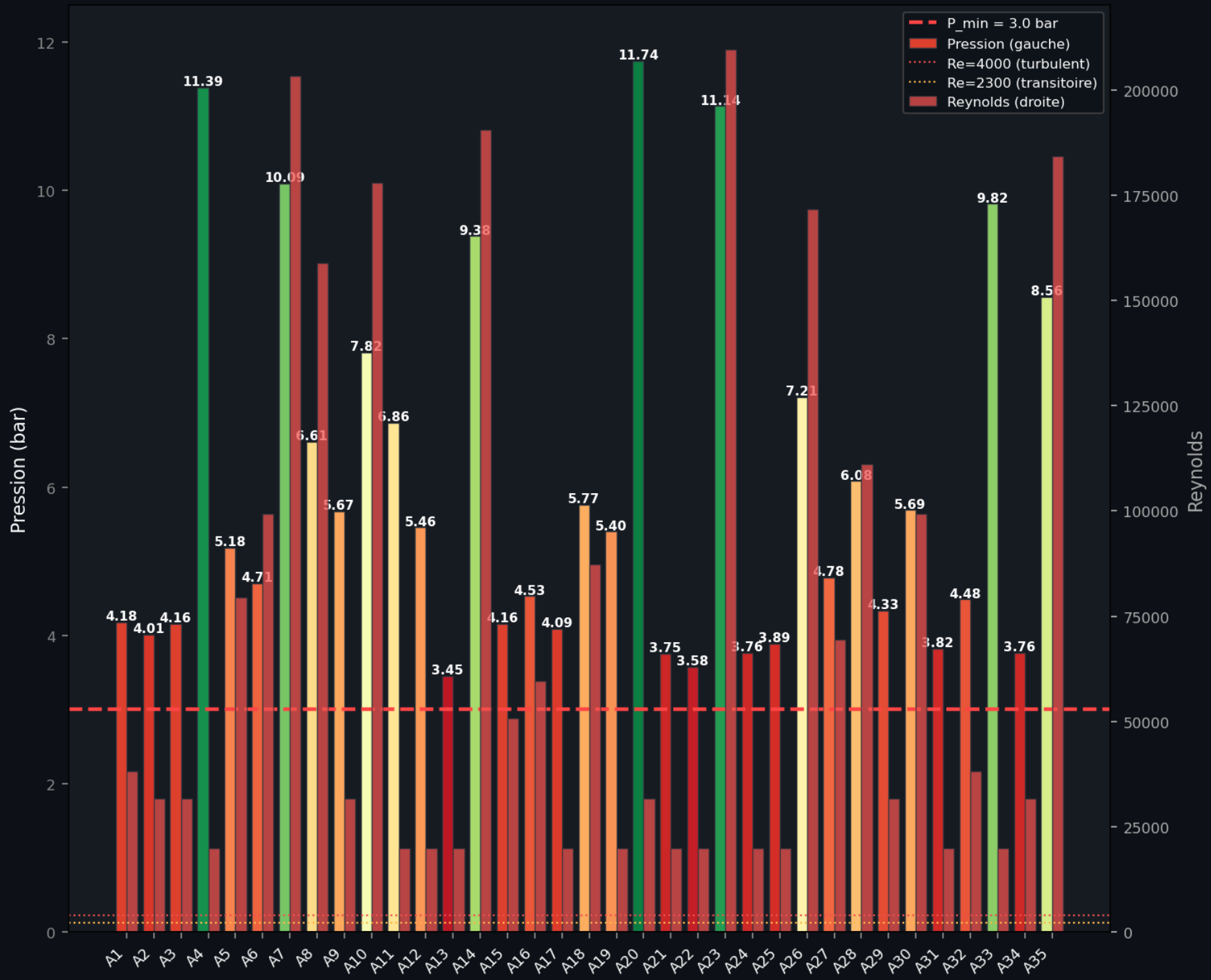
Pression + Reynolds par arroseur Bleu=laminaire Orange=transitoire Rouge=turbulent
