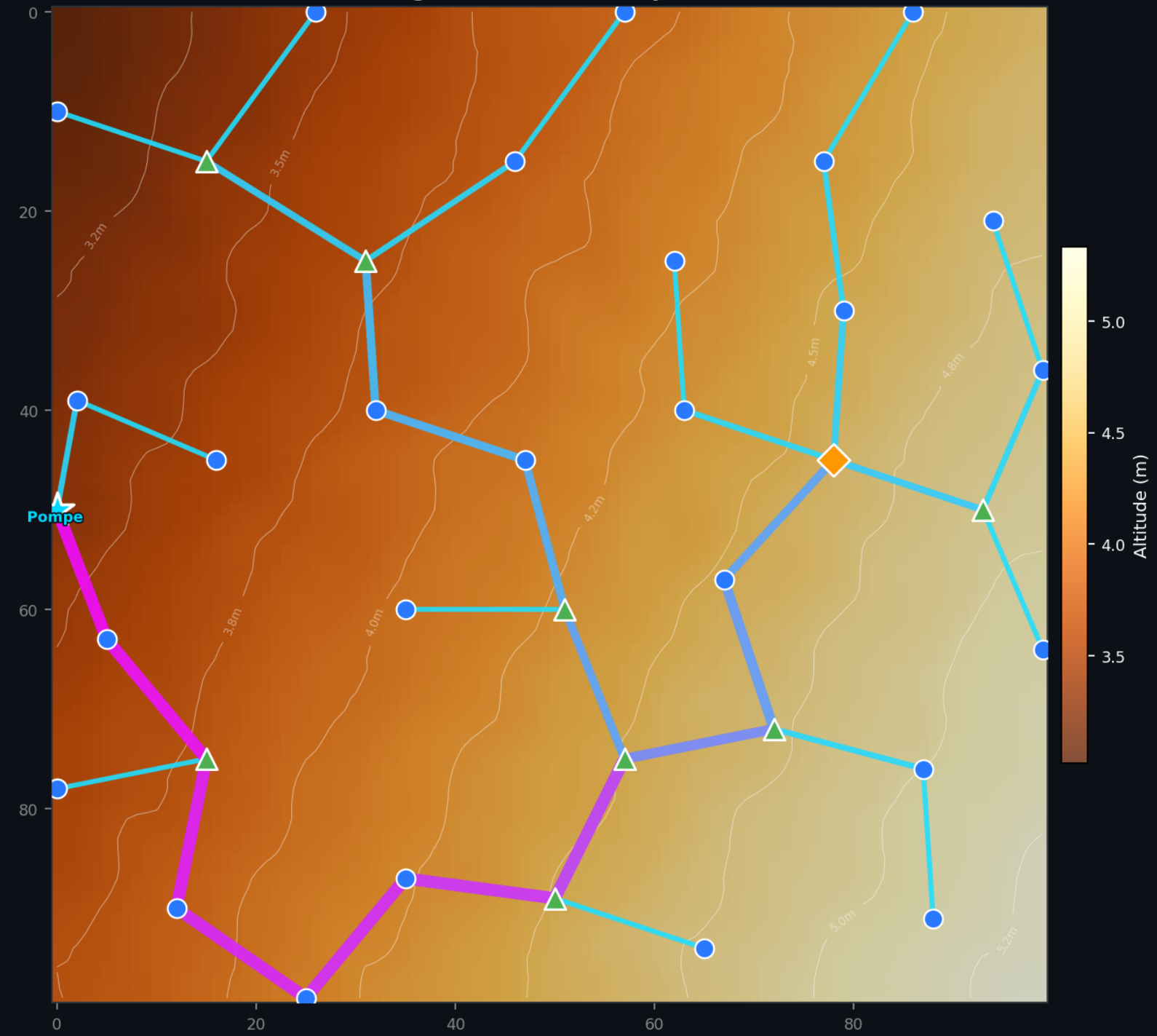
Relief — 200x200 m Lignes de niveau + tuyaux
