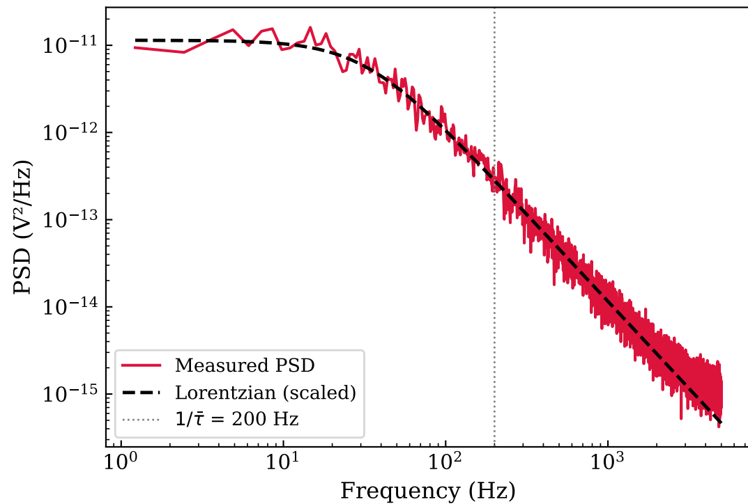
RTN Lorentzian PSD
