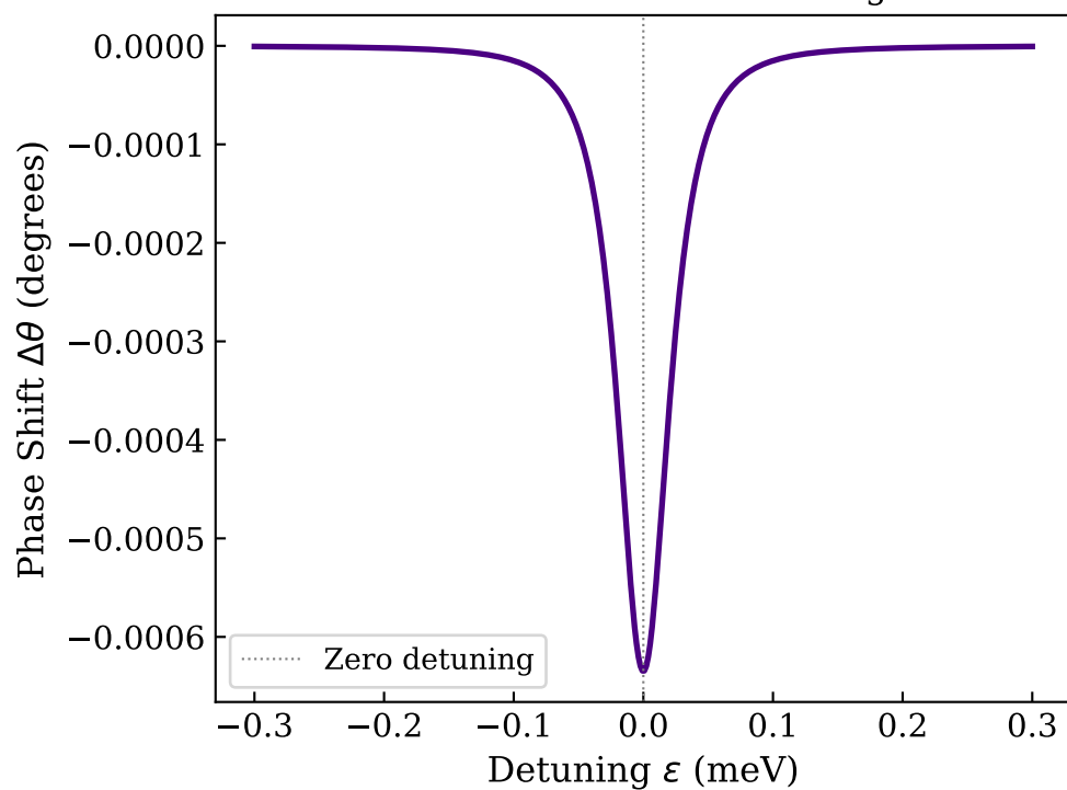
RF Phase Shift vs Detuning
