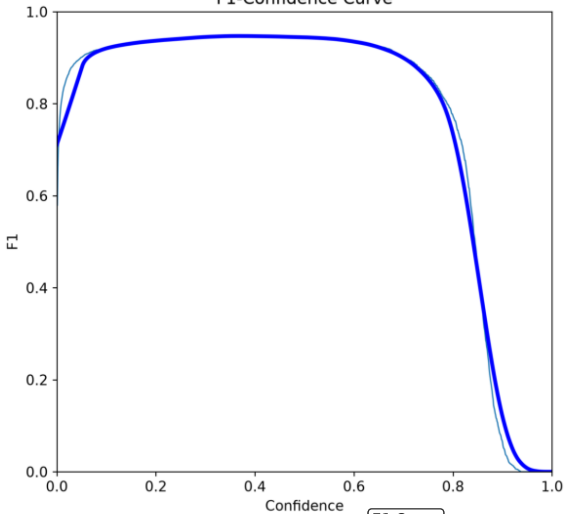
F1 Curve
