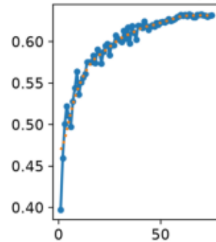
metrics/mAP50-95(B)
