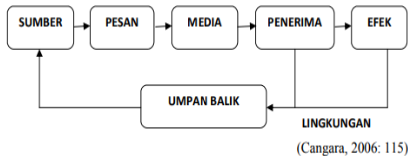
Gambar 2. 1 Unsur-unsur Komunikasi
