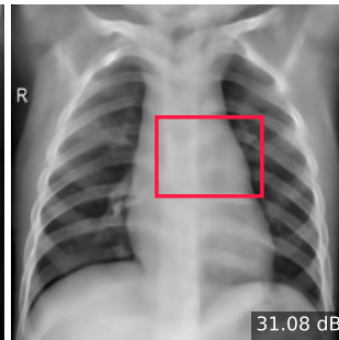
DnCNN
