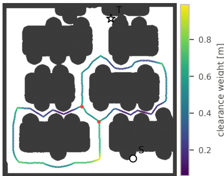
(d) weighted skeleton and nodes
