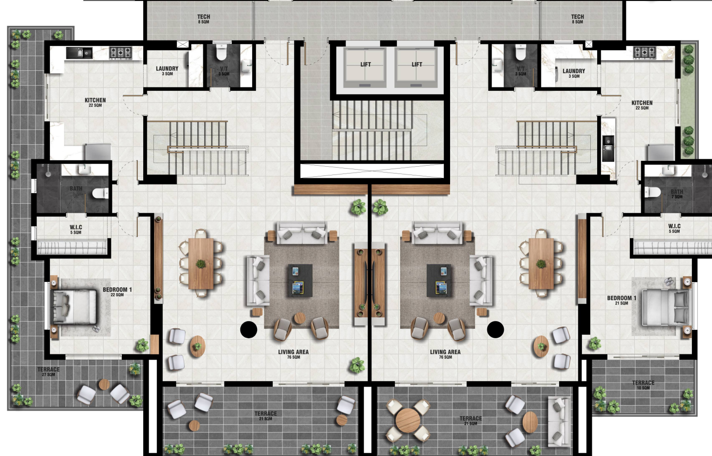
Duplex 3 4 Bedroom 217 sqm
