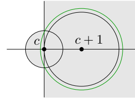
Figura 1.1: La zona pintada de gris és la zona en que F és holomorfa.
