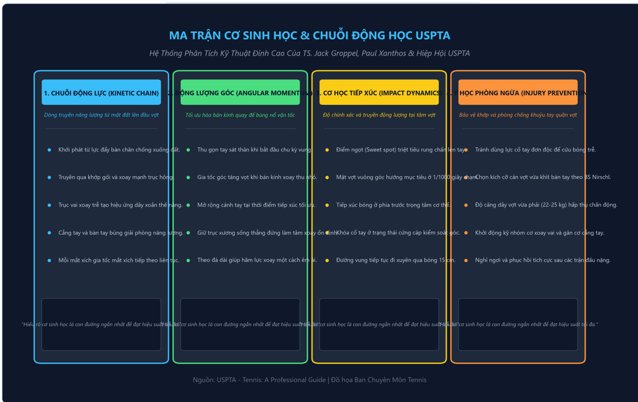
Sơ đồ 1: Chuỗi động lực tuyến tính, định luật bảo toàn mô-men động lượng và cơ học tiếp xúc bóng theo TS. Jack Groppel.
