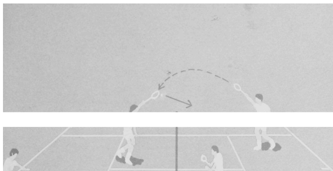
Hình 3-19. Khi đồng đội của người giao bóng đoán đúng, anh ta có thể lùi về để đón hầu hết bóng bổng trong nửa sân của mình.
