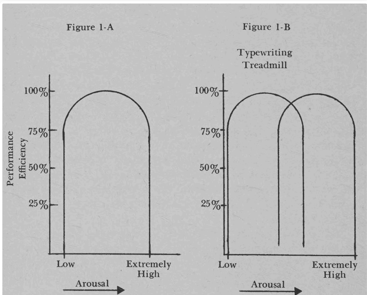
Hình 1-A và 1-B: tương quan giữa mức hưng phấn sinh lý (arousal) và hiệu suất thi đấu, với hai đường cong khác nhau cho hai loại nhiệm vụ (đánh máy và chạy máy tập).
