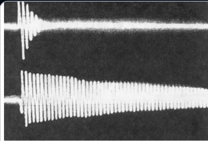
Hình 10: Biểu đồ dạng sóng dao động khung vợt ghi nhận trên máy hiện sóng: Sóng dao động tự do kéo dài (bên dưới) đối chiếu với sóng dao động bị hấp thụ triệt tiêu thần tốc chỉ sau 40–50 mili-giây (bên trên) nhờ áp lực kẹp tay cầm hợp lý.
