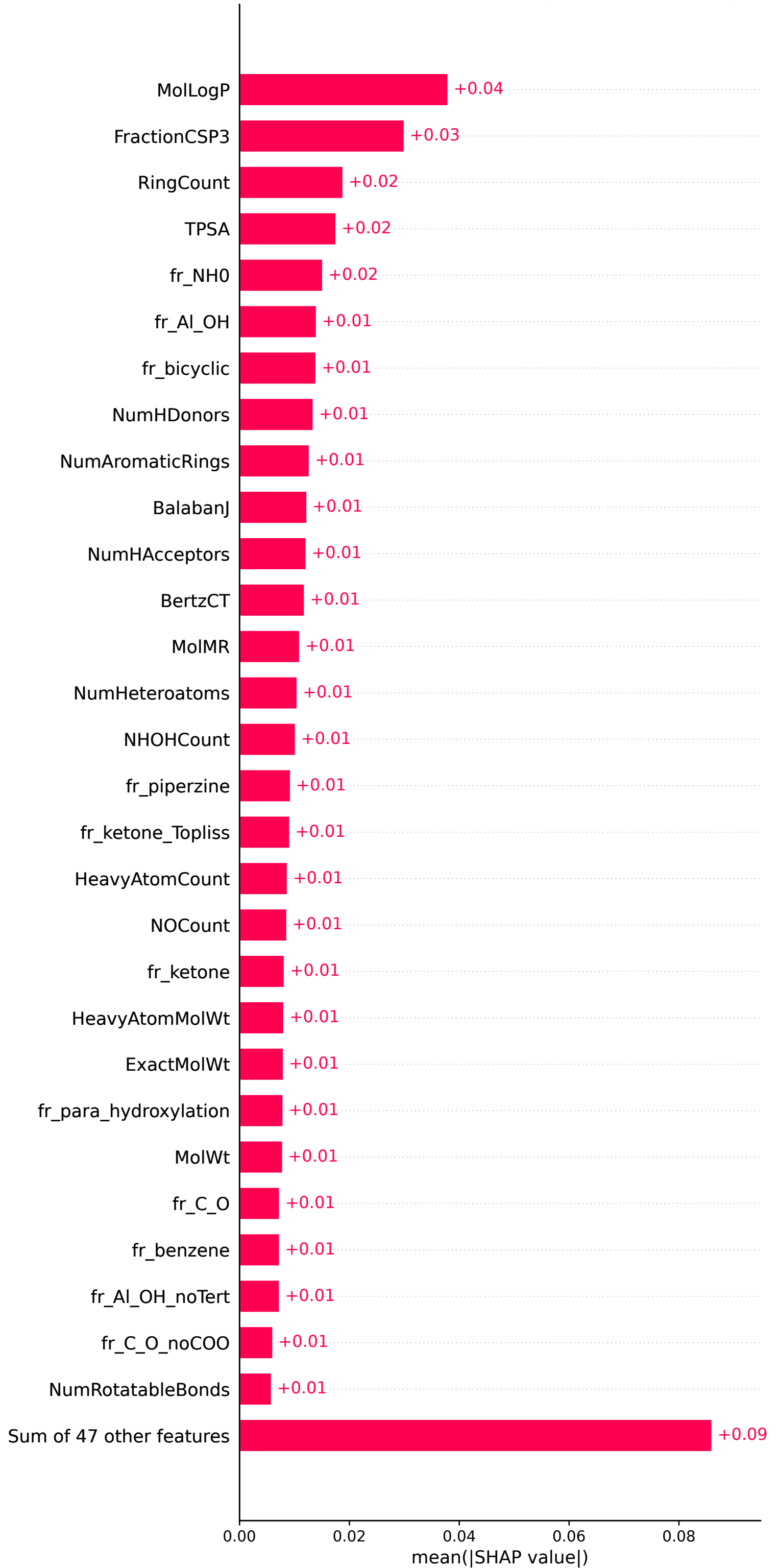
Mean absolute SHAP values for interpretable RDKit descriptors
