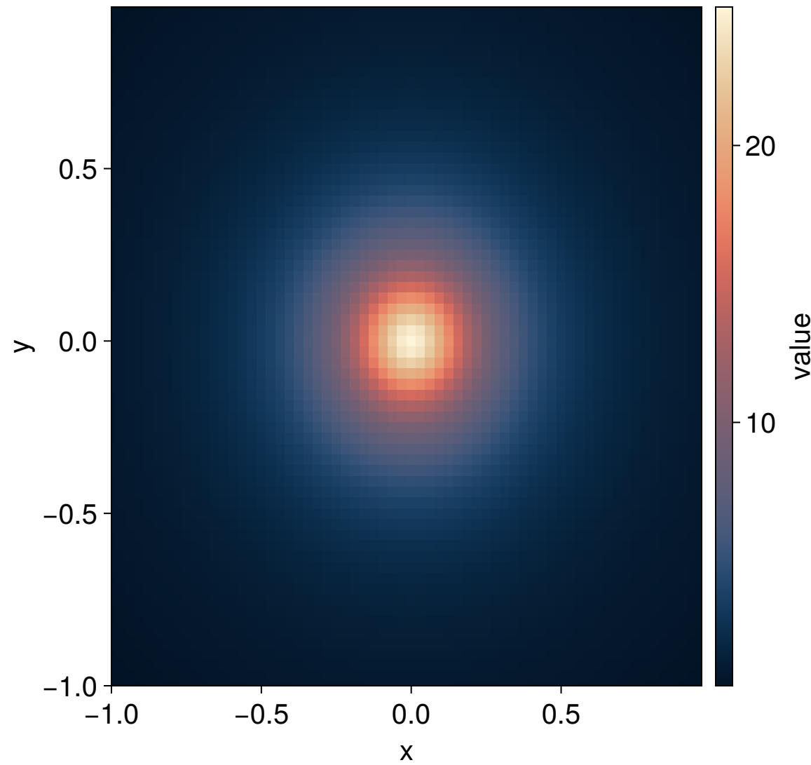
multiscale QTT
