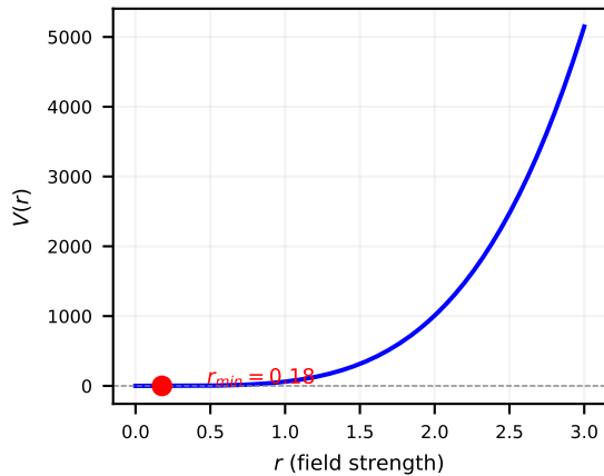
Cartan h_1
