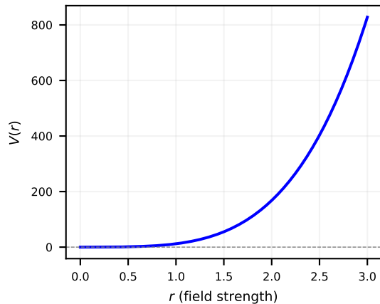
Cartan h_1
