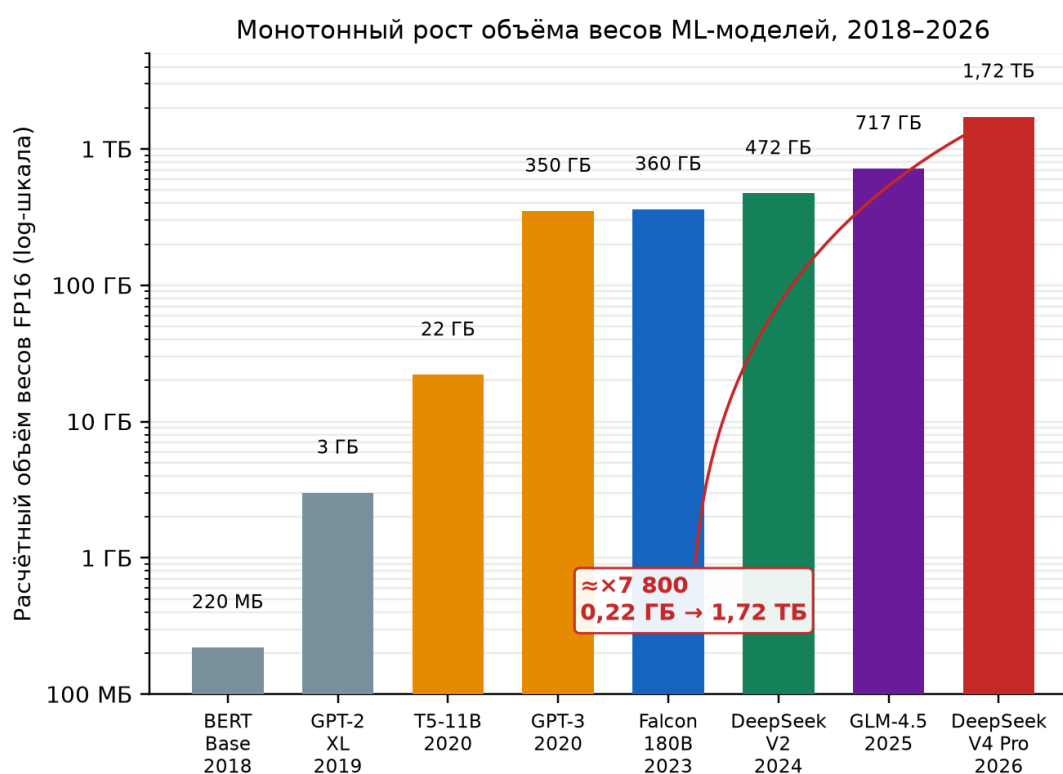
Рисунок 1 – Монотонная последовательность отобранных ML-моделей с возрастающим расчётным объёмом основных весов в FP16, 2018–2026 (логарифмическая шкала). График иллюстрирует рост выбранной последовательности, а не утверждает, что каждый выпуск соответствующего года крупнее всех других моделей.
