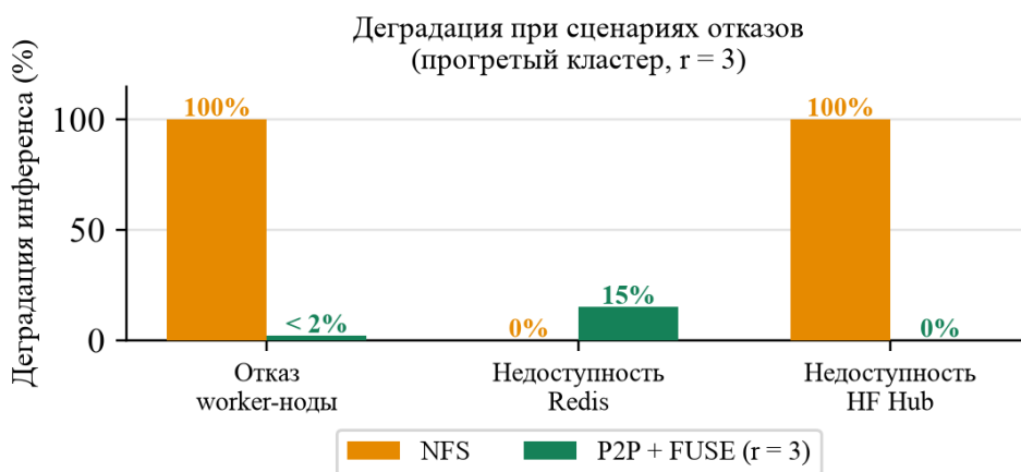
Рисунок 12 – Деградация инференса при трёх сценариях отказов (прогретый кластер, r = 3 ). NFS полностью теряет доступ при отказе сервера или HF Hub; P2P/FUSE деградирует до 15% при недоступности Redis и остаётся полностью работоспособен при сбое HF Hub.
