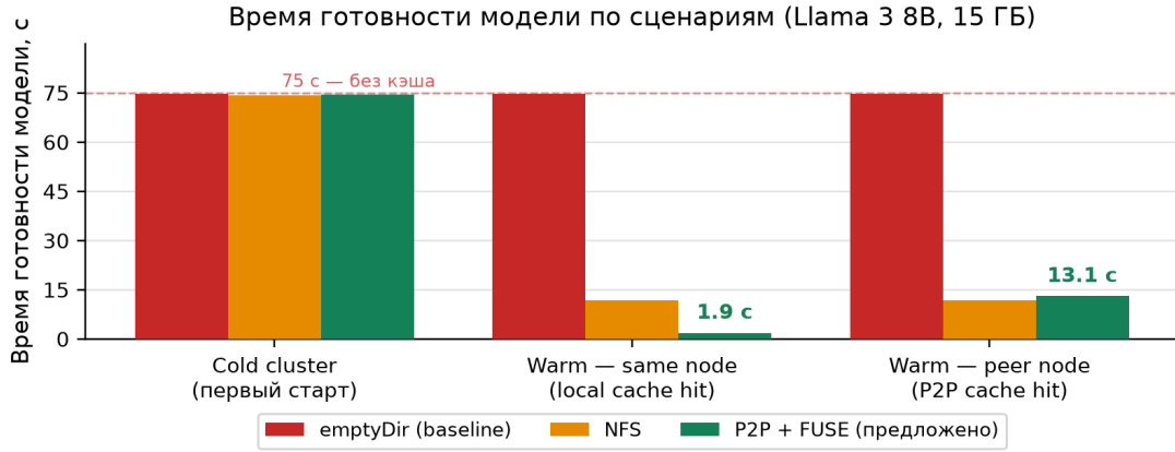
Рисунок 4 – Время готовности модели ( T_{\text{model\_ready}} ) по сценариям для Llama 3 8B (15 ГБ). При наличии локального кэша P2P/FUSE-подход обеспечивает T_{\text{model\_ready}} = 1.9 с против 74.8 с у baseline.
