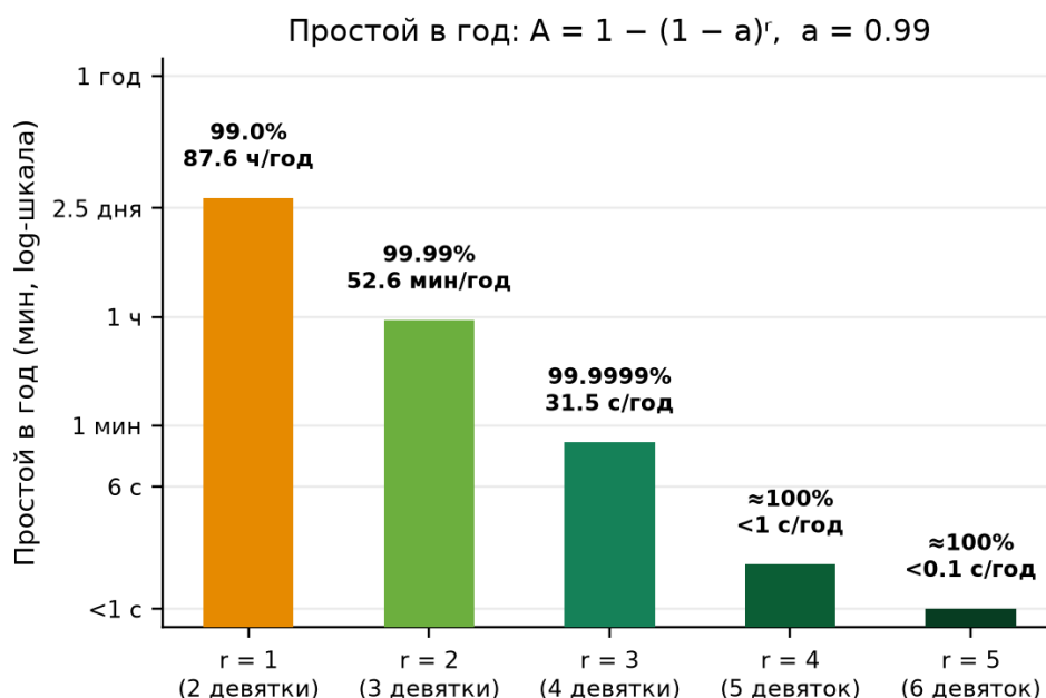
Рисунок 3 – Простой в год в зависимости от коэффициента репликации чанков ( a = 0.99 ). При r = 3 простой сокращается с 87.6 ч/год до 31.5 с/год — переход от двух к четырём девяткам доступности.
