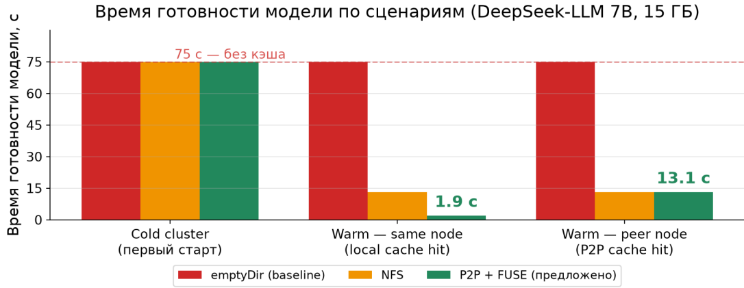
Рисунок 6 – Время готовности модели ( T_{\text{model\_ready}} ) по сценариям для DeepSeek-LLM 7B (15 ГБ). При наличии локального кэша P2P/FUSE-подход обеспечивает T_{\text{model\_ready}} = 1.9 с против 74.8 с у baseline.
