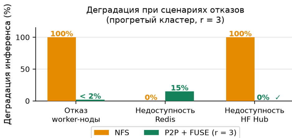
Рисунок 8 – Деградация инференса при трёх сценариях отказов (прогретый кластер, r = 3 ). NFS полностью теряет доступ при отказе сервера или HF Hub; P2P/FUSE деградирует до 15% при недоступности Redis и остаётся полностью работоспособен при сбое HF Hub.
