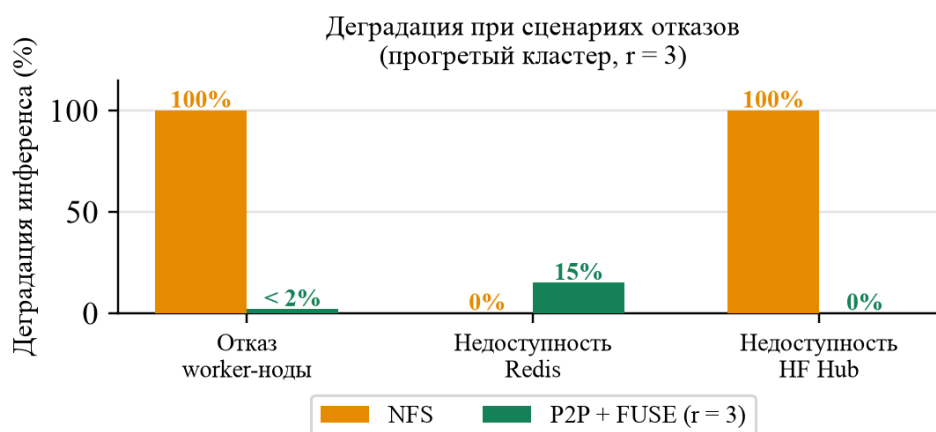
Рисунок 11 – Деградация инференса при трёх сценариях отказов (прогретый кластер, r = 3 ). NFS полностью теряет доступ при отказе сервера или HF Hub; P2P/FUSE деградирует до 15% при недоступности Redis и остаётся полностью работоспособен при сбое HF Hub.
