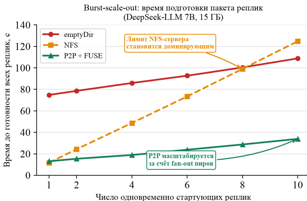
Рисунок 9 – Время подготовки burst-пакета из N реплик в прогретом кластере (DeepSeek-LLM 7B, 15 ГБ). Для emptyDir прогрев кластера не даёт выигрыша, NFS упирается в пропускную способность одного сервера, а P2P/FUSE распределяет нагрузку между несколькими нодами.
