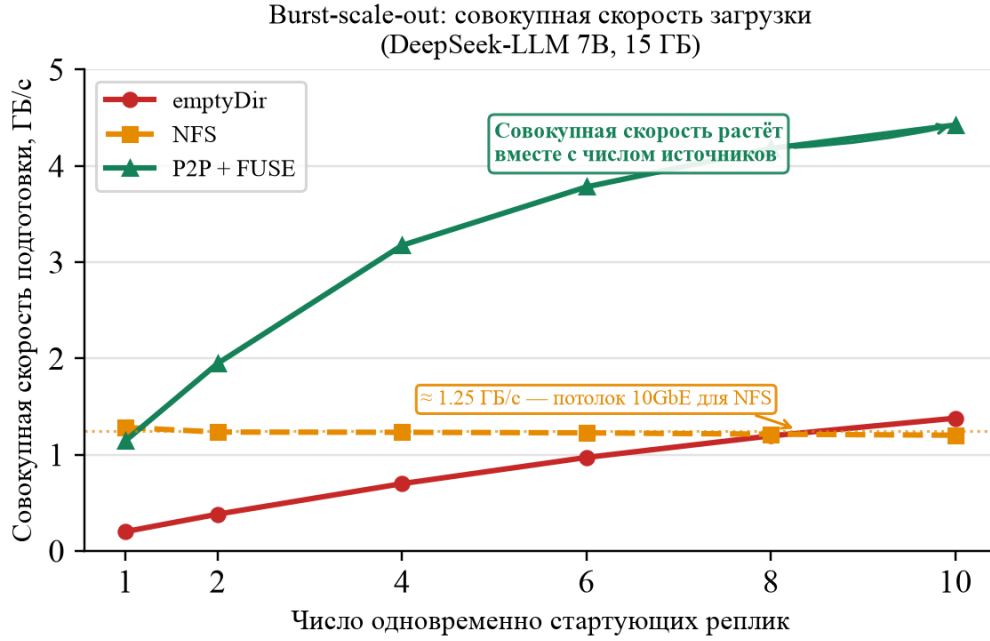
Рисунок 10 – Совокупная скорость подготовки N реплик в прогретом кластере (DeepSeek-LLM 7B, 15 ГБ). Для NFS наблюдается насыщение около пропускной способности 10GbE-сервера, тогда как P2P/FUSE увеличивает суммарную скорость за счёт fan-out между несколькими агентами и локальными дисками.
